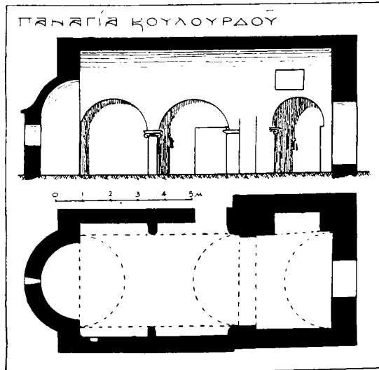
Εἰκ. 177. Κάτοψις ναοῦ Παναγίας Κουλουρδοῦς.
