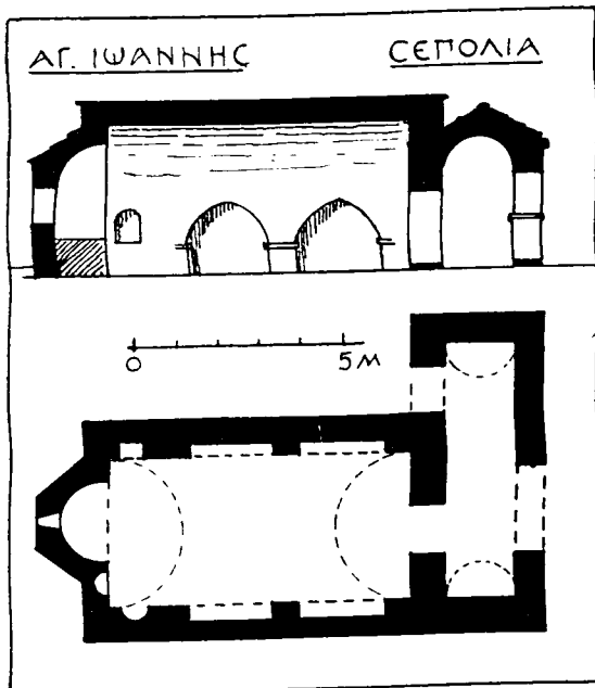
Εἰκ. 179. Κάτοψις καὶ τομὴ Ἀγ. Ἰωάννου Σεπολίων.
