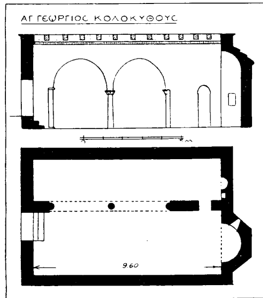
Εἰκ. 178. Κάτοψις καὶ τομὴ Ἀγ. Γεωργίου.
