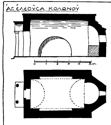
Εἰκ. 180. Κάτοψις καὶ τομὴ Ἀγ. Ἐλεούσης.
